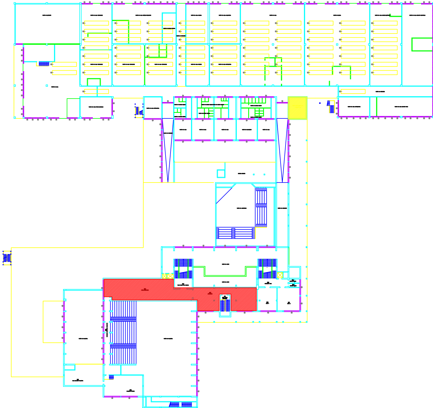
PIANTA PIANO AMMEZZATO
